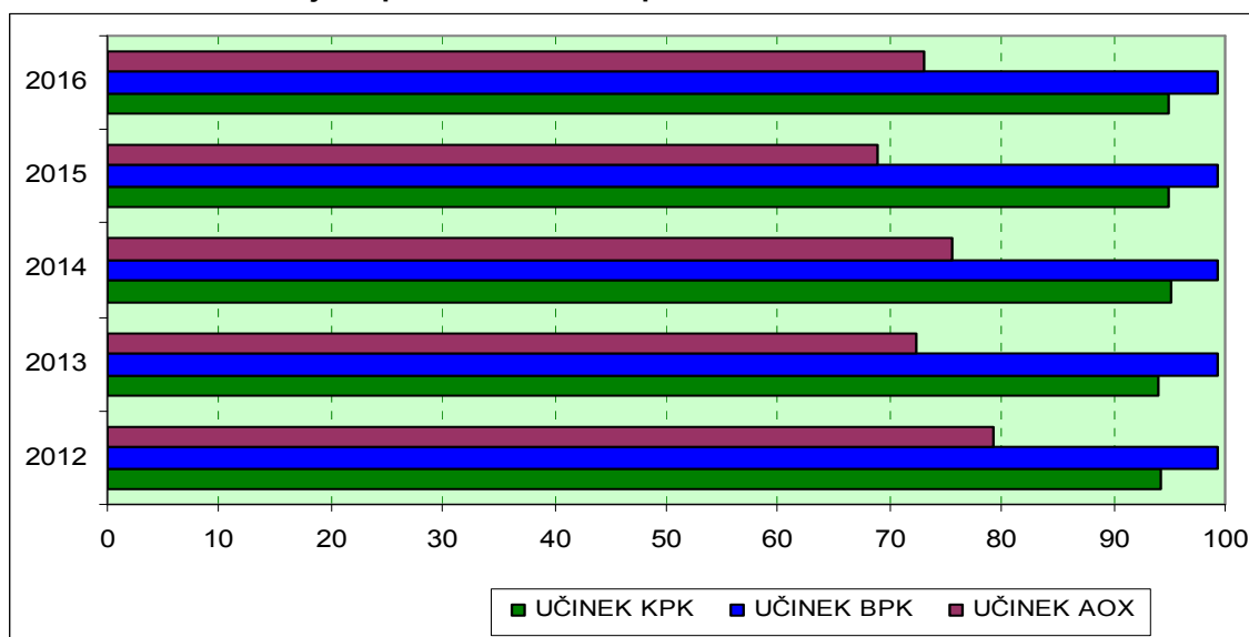
GRAF 1: Učinki čiščenja odpadnih vod na skupni ČN VIPAP
