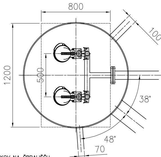
SHEMA PRIKLJUČKOV NA ČRPALIŠČU
