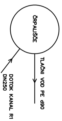
SCHEMA PRIKLJUČKOV NA ČRPALIŠČU
