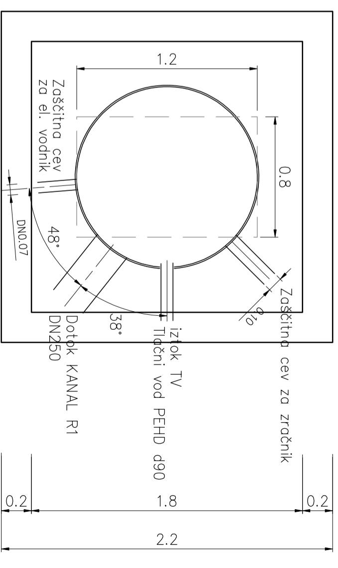
SCHEMA PRIKLJUČKOV NA ČRPALIŠČU
